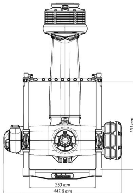
PAN Flanges
